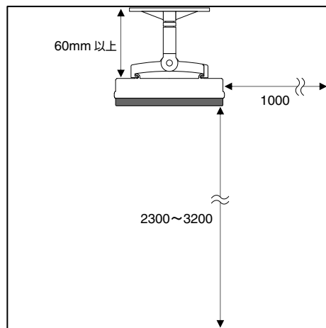
【天井取り付け】天井と平行（側面）
