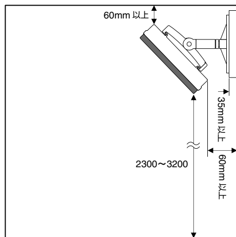
【壁取り付け】角度付（側面）
